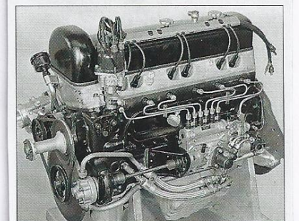
De motor leverde dankzij directe (!) brandstofinjectie meer vermogen dan de racer met carburateurmotor
